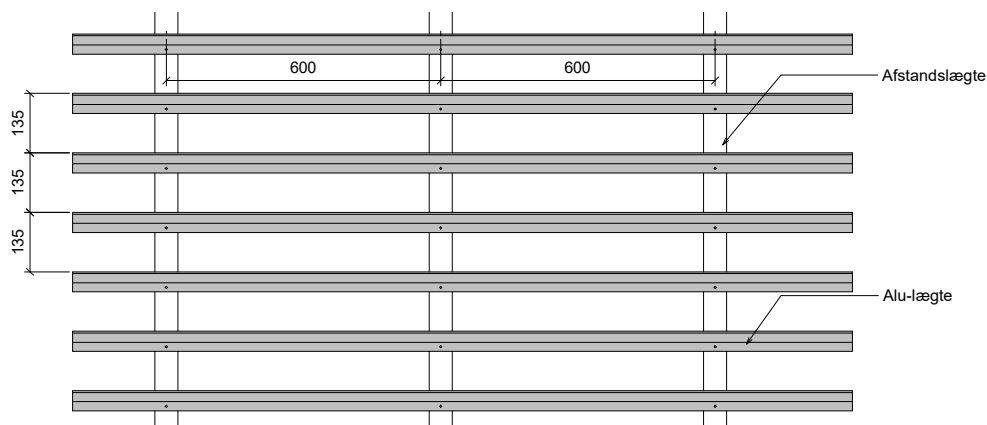
Figur 5 Udsnit af opstalt af afstandslægter samt alu-lægterne.
