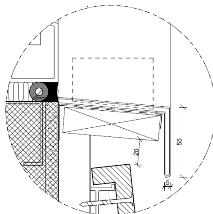
Figur 15 Vertikalt snit gennem PTK alu-inddækningsprofil, bund
