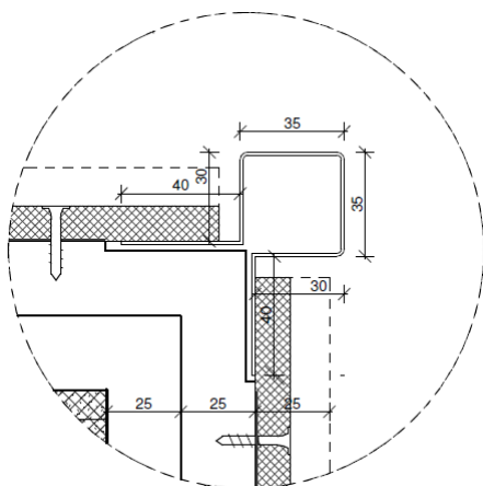
Figur 11 Horizontalt snit gennem PTK alu-hjørneprofil type 2, 75x75mm
