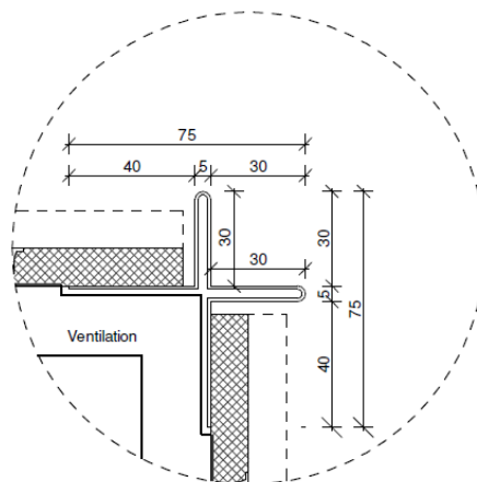
Figur 12 Horizontalt snit gennem PTK alu-hjørneprofil type 3, 75x75mm
