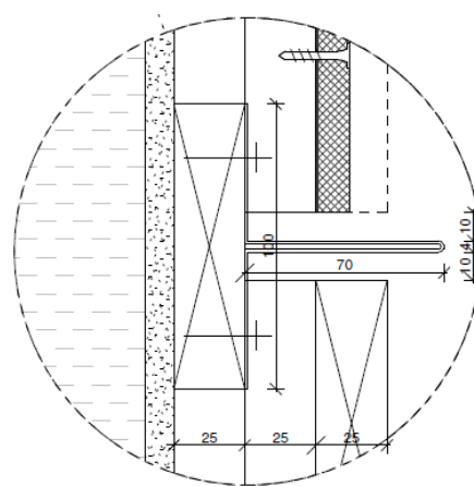
Figur 14 Horizontalt snit gennem PTK alu-inddækningsprofil
